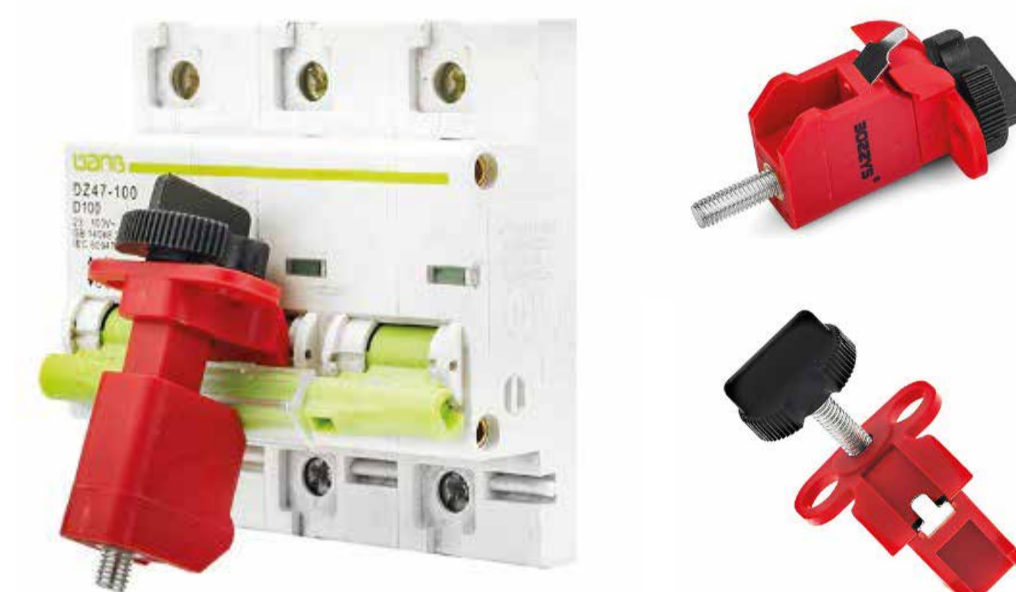
bloqueo de barra de unión BYBDD003
